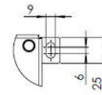
DETAIL A MA8TAB 2 : 5
